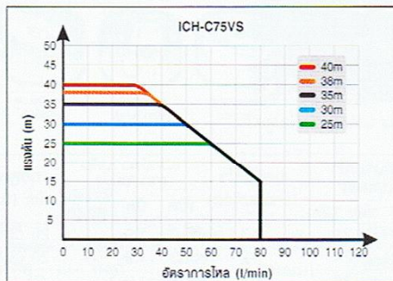
PERFORMANCE CURVE : สำหรับ ICH
