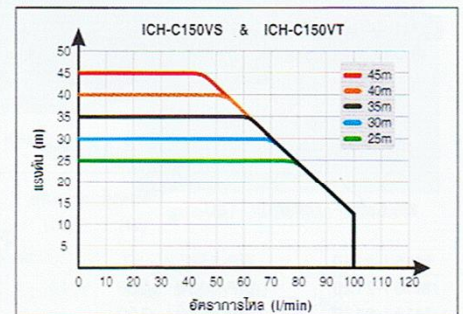
PERFORMANCE CURVE : สำหรับ ICH
